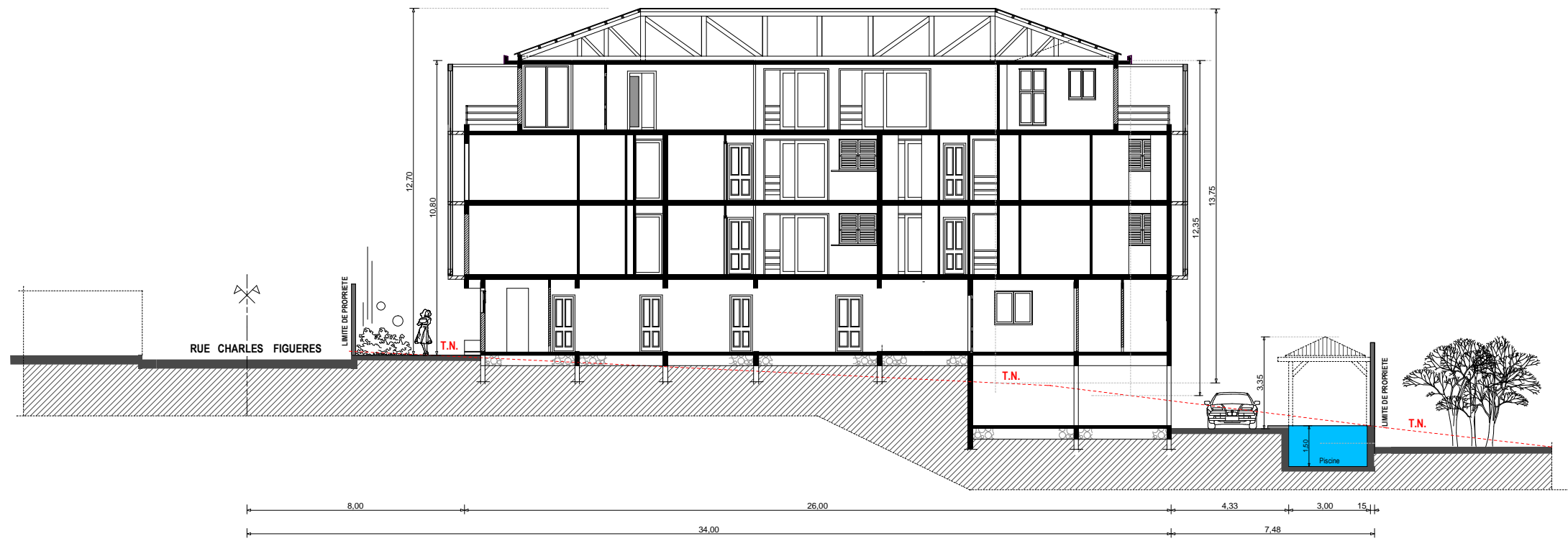
COUPE SUR PROFIL TERRAIN ECHELLE 1/200ème
